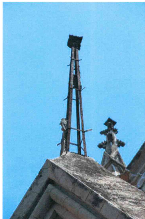
Pináculo de argamassa armada com perda de elementos
