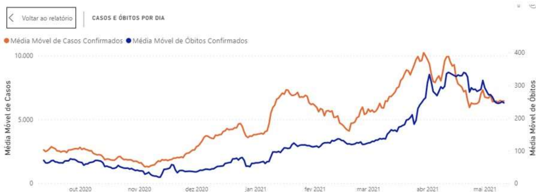
Figura 4 – Média móvel de casos confirmados (alaranjado), óbitos por data de ocorrência (azul escuro) e óbitos por data de notificação (azul claro). Minas Gerais, 2020 e 2021.
